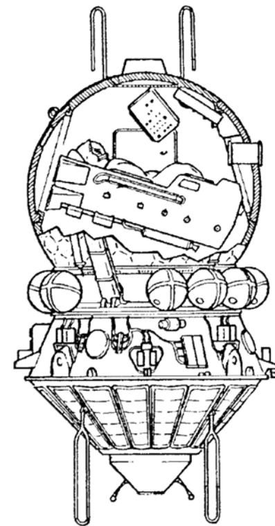
Γραμμικό σχέδιο της διαστημοσκευής Vostok .
